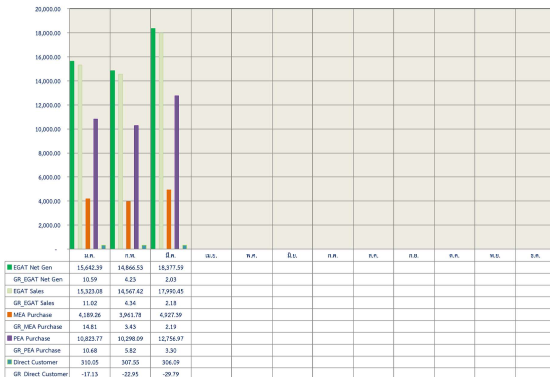
หน่วยผลิตไฟฟ้าสุทธิ และหน่วยจำหน่าย กฟผ. รายเดือน ประจำปี 2565 (ล้านหน่วย)
